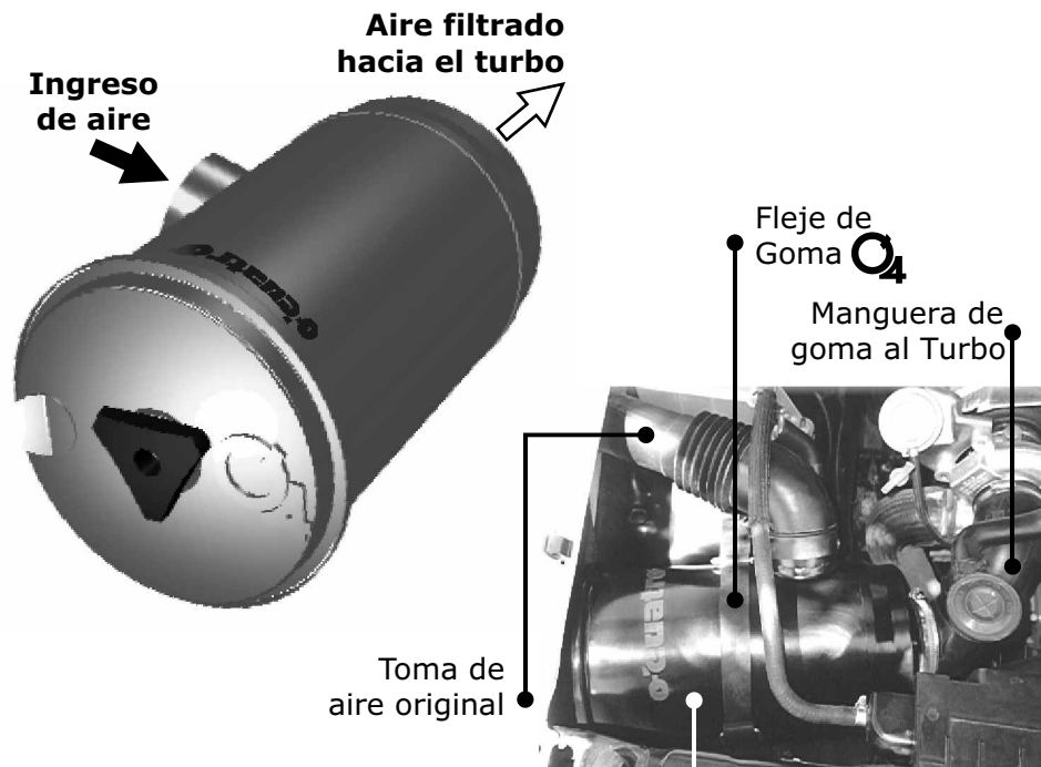
Carcasa O 4 Modelo SS 116 CH Elemento Filtrante E 116
